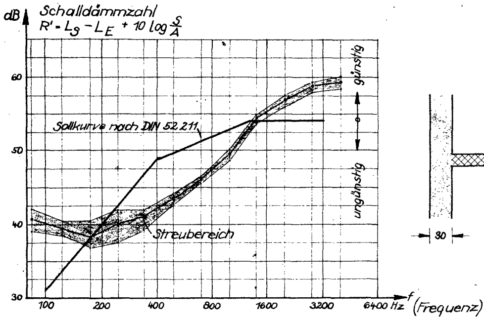
Hochlochziegel B, 1, 2/150, 240x175x155 nach DIN 105
