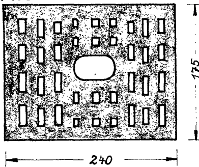
Hochlochziegel B, 1, 2/150, 240x175x155 nach DIN 105
